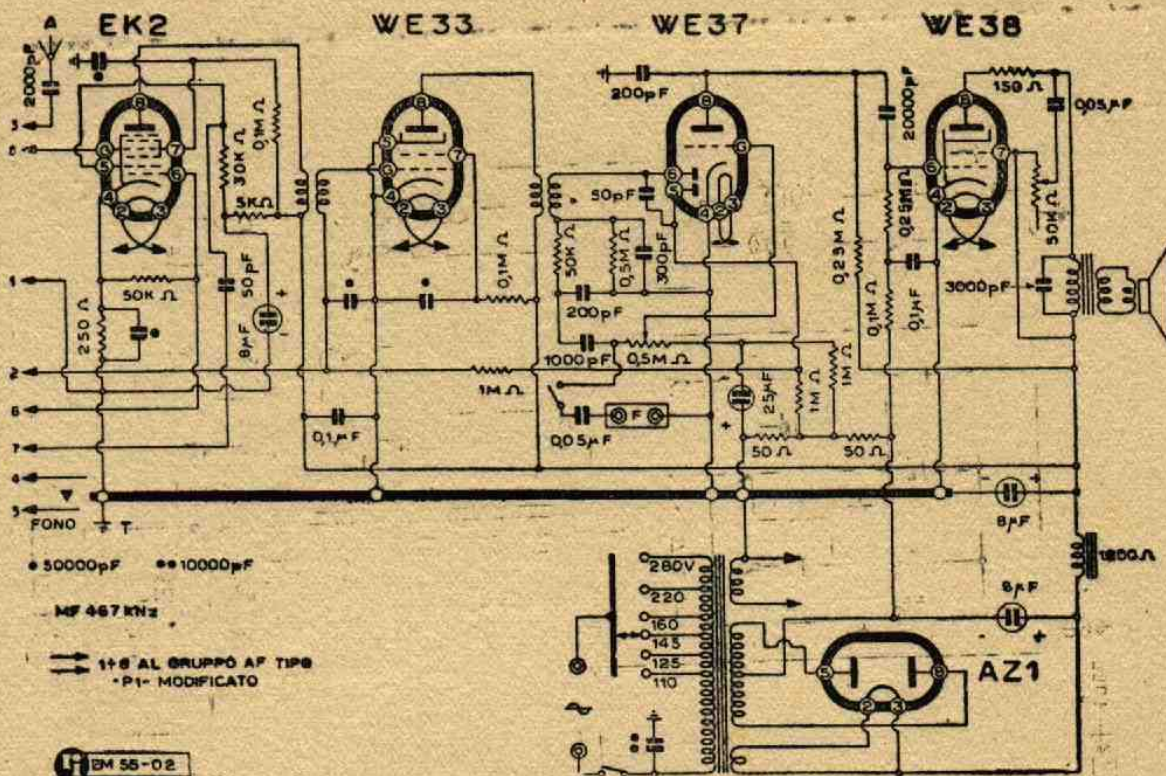
Lo schema elettrico del mod. 556.
