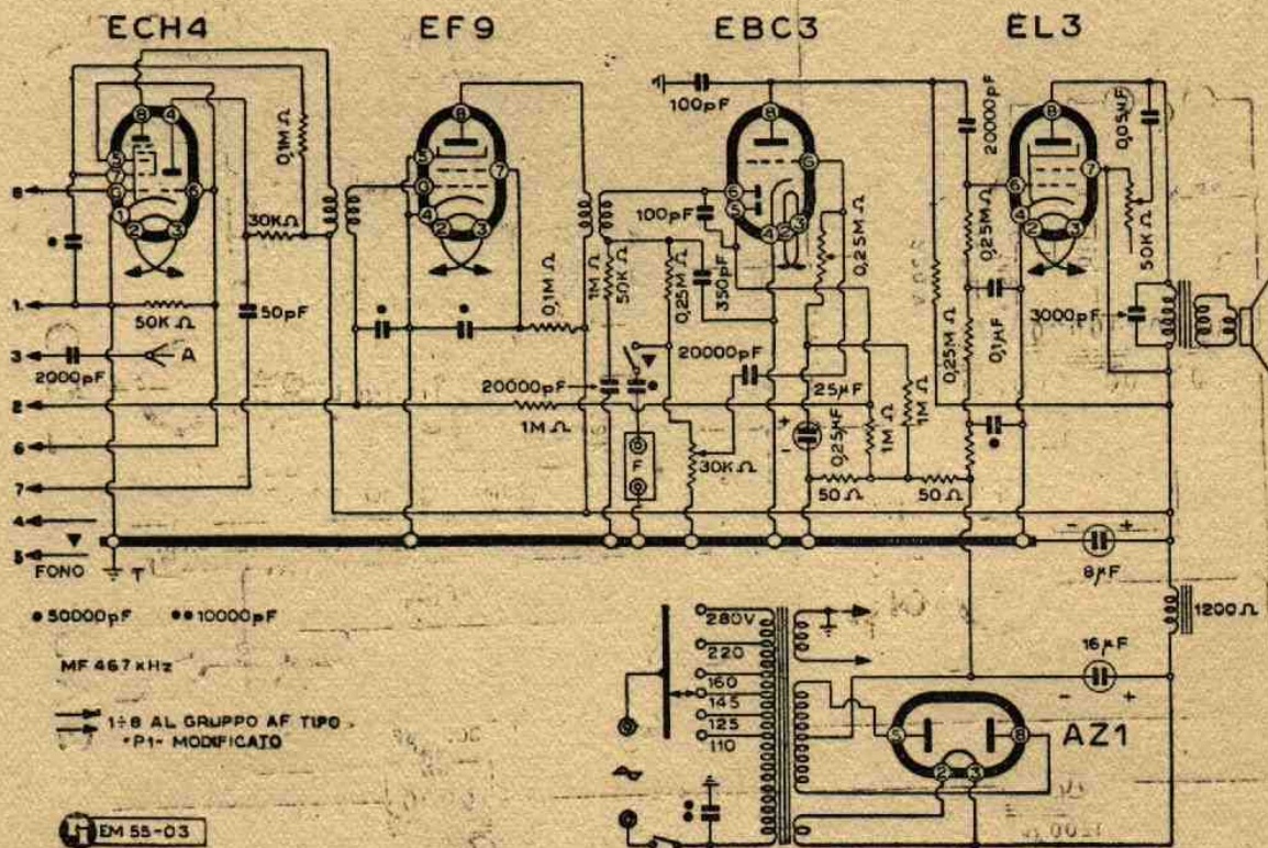
Lo schema elettrico del mod. 556 L.
